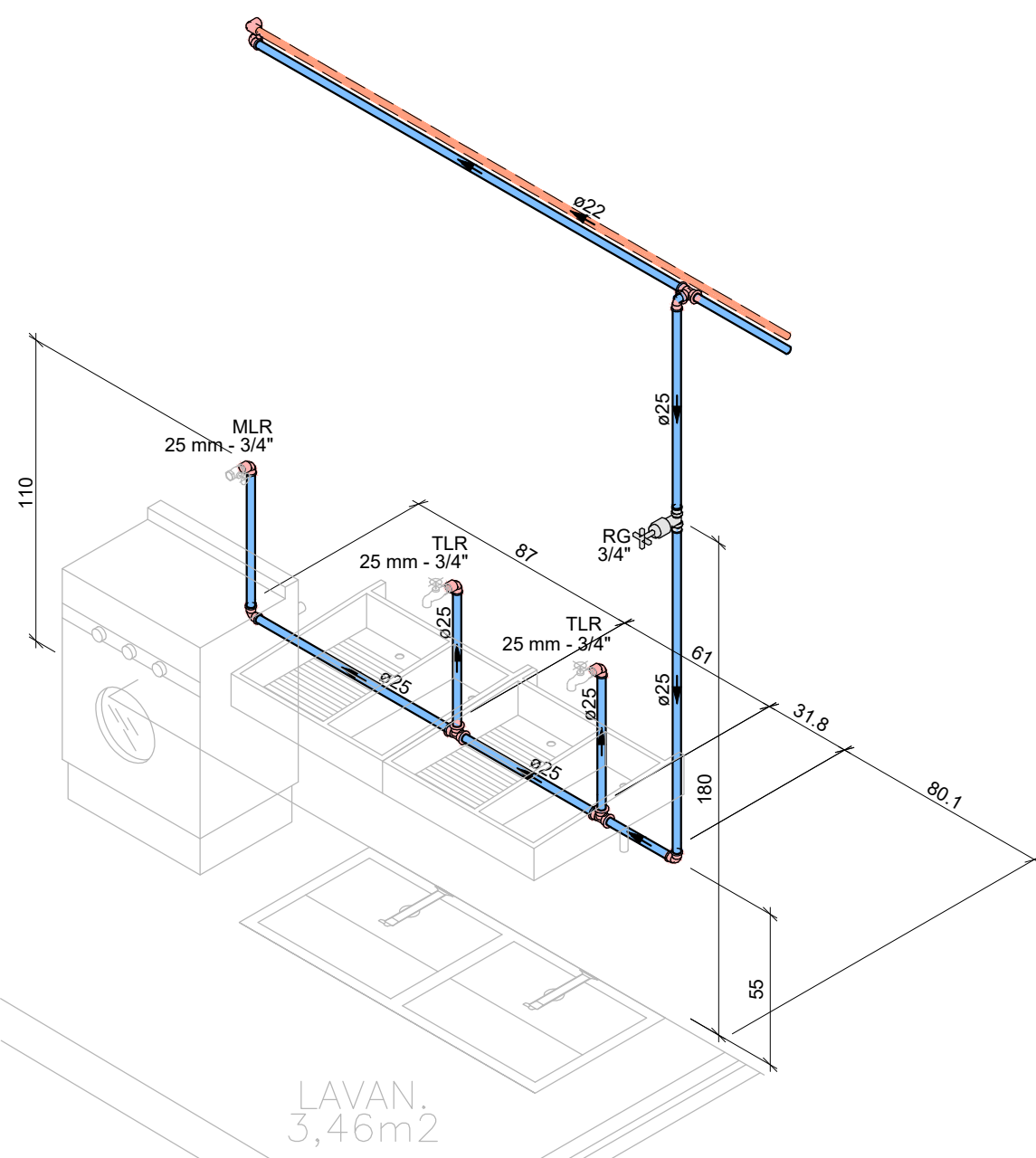
Detalhe HI-4 1 : 25
